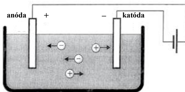
Obr. 11.3 Schéma elektrolyzy
