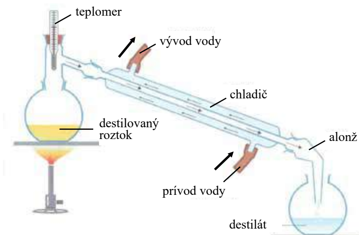
Obr. 2.15 Schéma destilačnej aparatury
