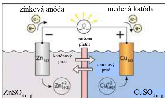
Obr. 11.6 Daniellov článok
