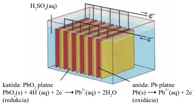
Obr. 11.8 Schéma oloveného akumulátora a zápis redoxných dejov na elektródach pri jeho vybíjaní
