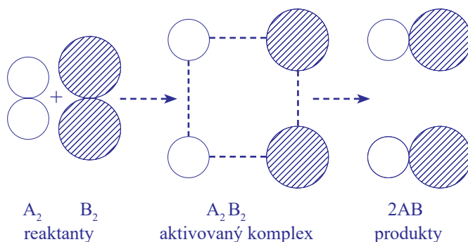
Obr. 9.3 Schéma reakcie A_2 + B_2 \longrightarrow 2AB
