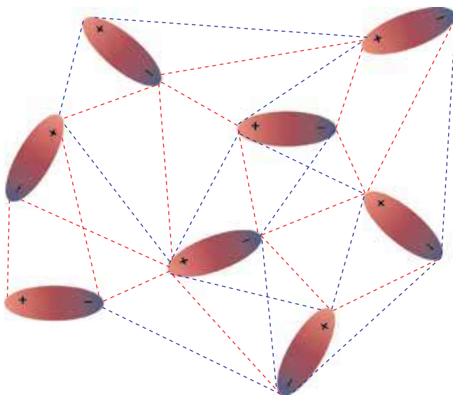
Obr. 6.10 Vzájomné pôsobenie medzi polárnymi molekulami
