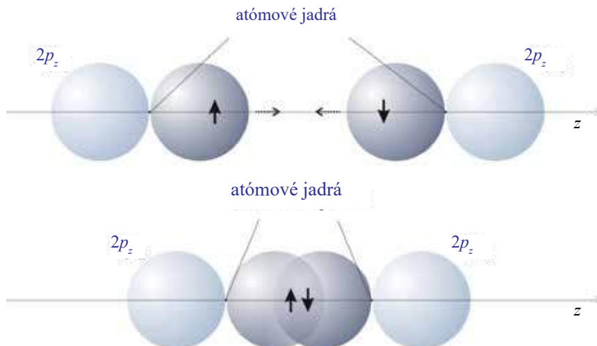
Obr. 6.4 Prekryv 2p_z orbitálov atómov fluóru pri vzniku \sigma väzby
