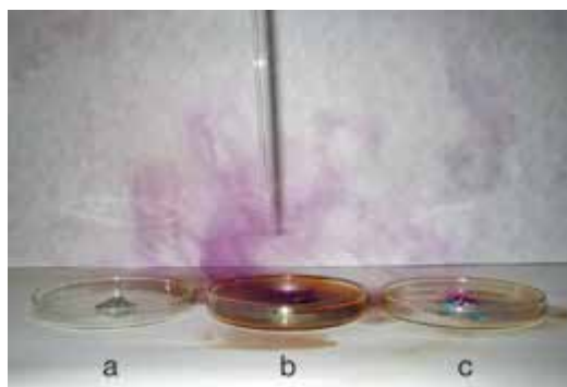
Obr. 9.8 Chemická reakcia hliníka s jódom v prítomnosti H_2O ako katalyzátora
