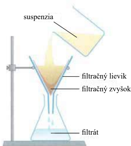
Obr. 2.2 Schéma filtračnej aparatury
