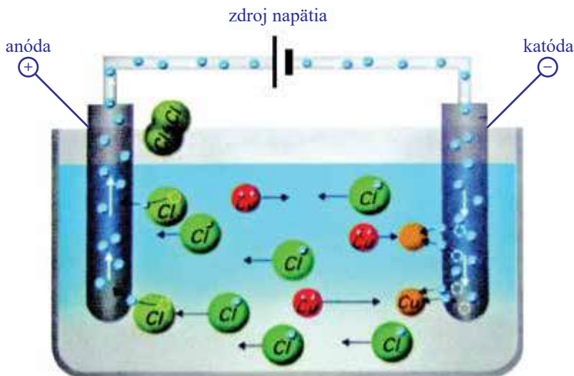
Obr. 11.4 Elektrolýza \text{CuCl}_2
