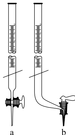
Obr. 12.9 Byrety a – s rovným kohútom b – s bočným kohútom
