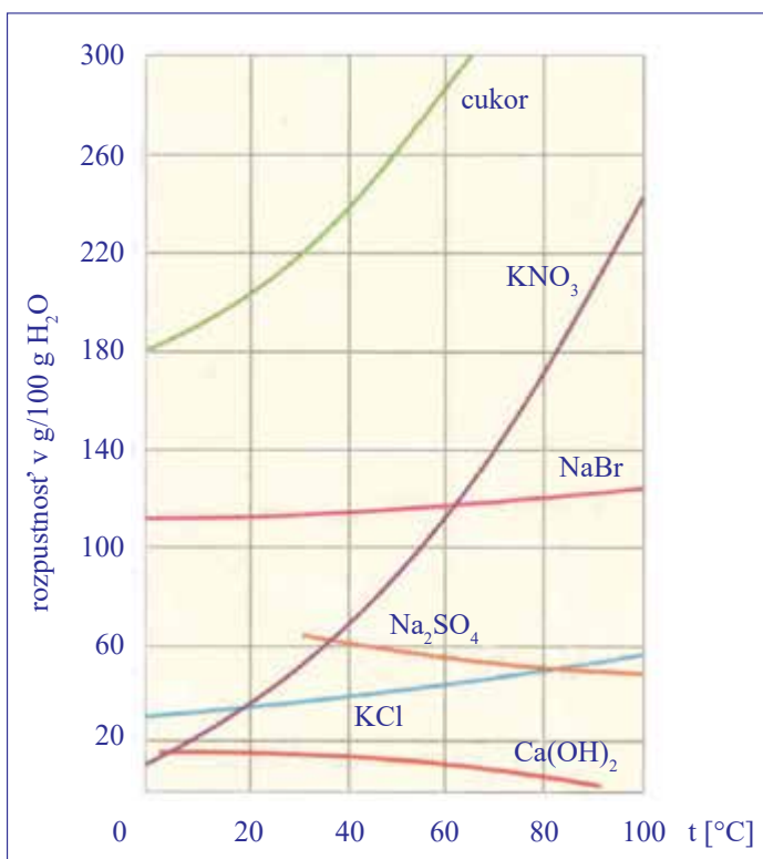
Obr. 2.20 Krivky rozpustnosti vybraných látok
