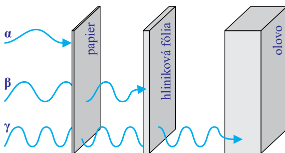
Obr. 3.3 Prenikavosť žiarenia \alpha , \beta , \gamma
