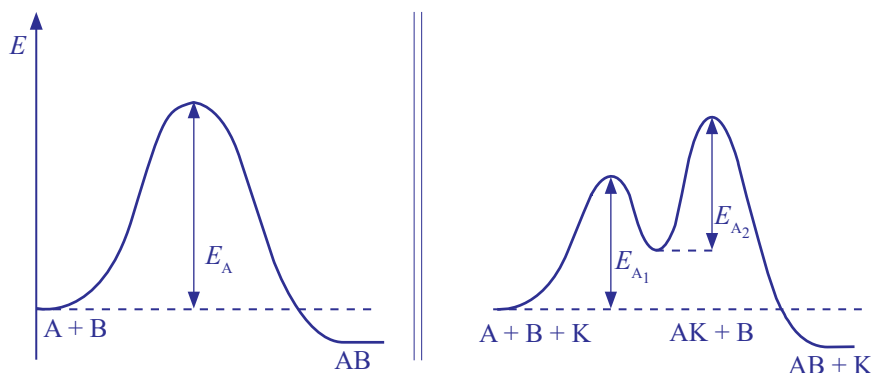
Obr. 9.9 Energetické zmeny látok pri nekatalyzovanej a katalyzovanej chemickej reakcii
