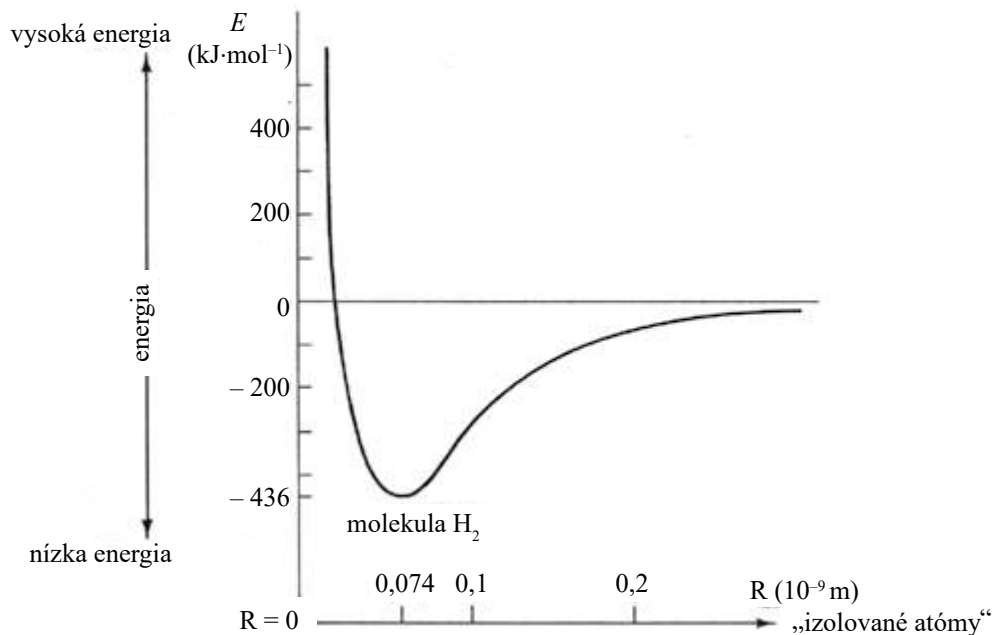
Obr. 6.1 Energetické zmeny pri približovaní sa dvoch atómov vodíka
