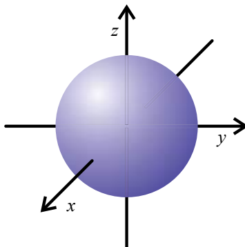
Obr. 3.5 Orbitál s
