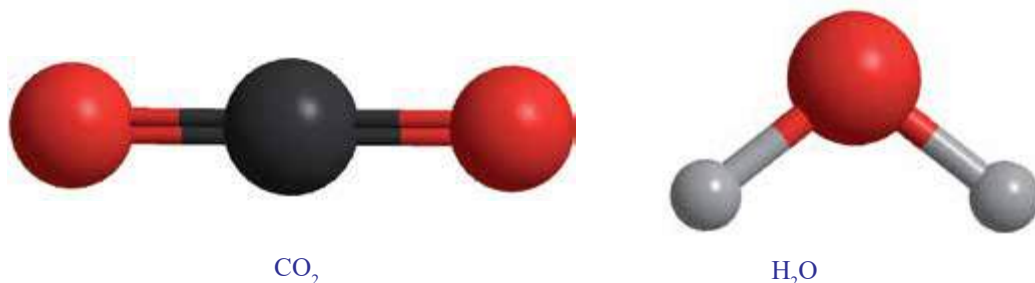
Obr. 6.6 Priestorové usporiadanie atómov v molekulách \text{CO}_2 a \text{H}_2\text{O}
