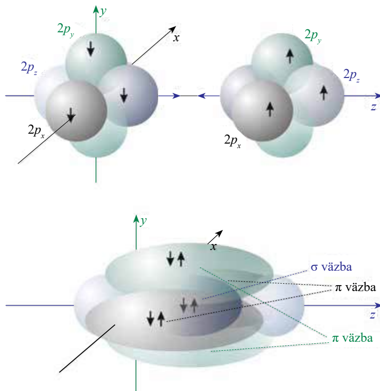
Obr. 6.5 Prekryv orbitálov 2p_x , 2p_y a 2p_z pri vzniku trojitej väzby v molekule dusíka
