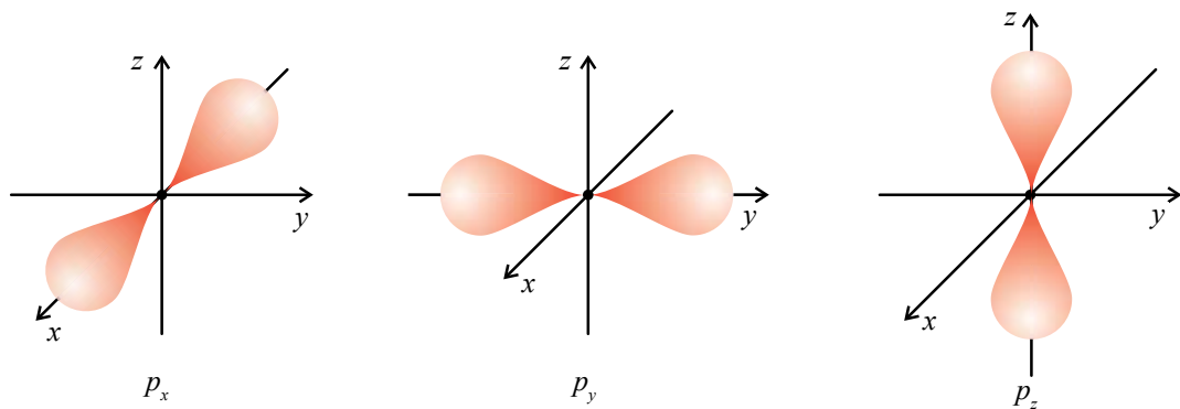
Obr. 3.6 Orbitály p_x, p_y, p_z
